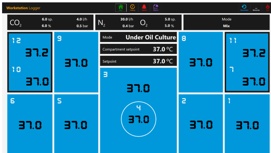
23.3 pav. Darbo stotelės duomenų registratoriaus rodinys normaliomis darbo sąlygomis (su dujų maišytuvu)
